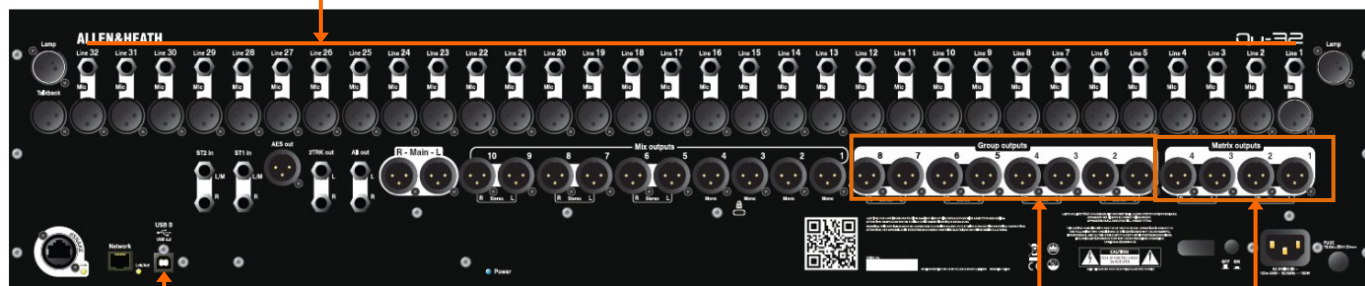
Qu-32 32 entrées micro/ligne
